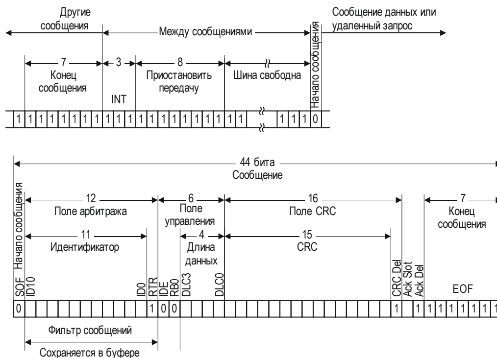
Рисунок 26.4 – Удаленный запрос данных (стандартный формат)
