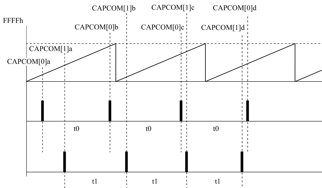
Рисунок 13.6 — Временные интервалы в непрерывном режиме
