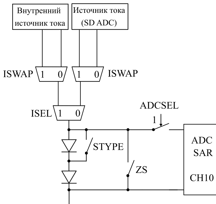
Рисунок 23.1 – Структурная схема датчика температуры
