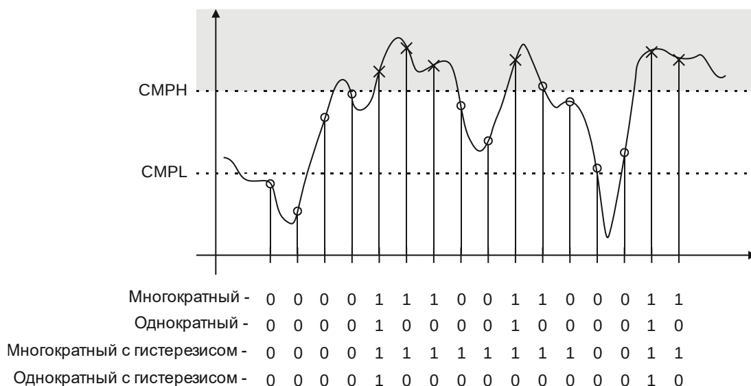
Рисунок 21.17 – Функционирование триггера при CTC = 10b
