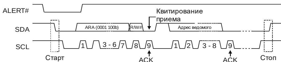
Рисунок 27.9 – Передача адреса отклика на сигнал предупреждения
