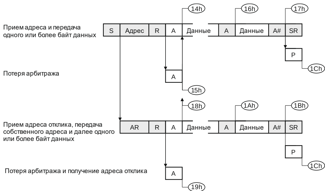
Рисунок 27.22 – Режим FS ведомого передатчика
