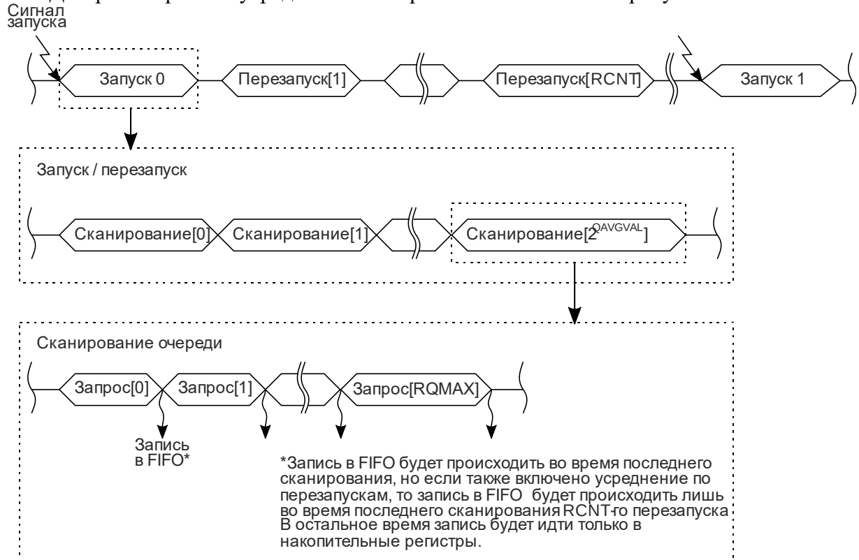
Рисунок 21.11 – Режим усреднения сканированием
