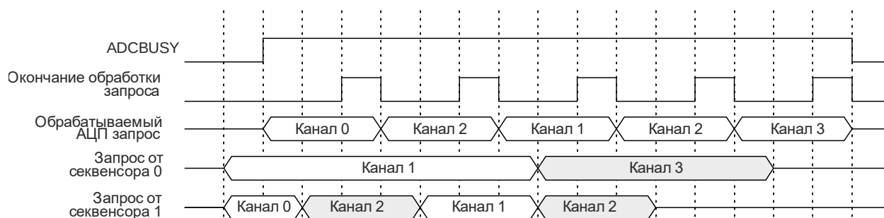
Рисунок 21.13 – Пример арбитража запросов, серым выделены запросы по каналам с установленным битом PRIORITY
