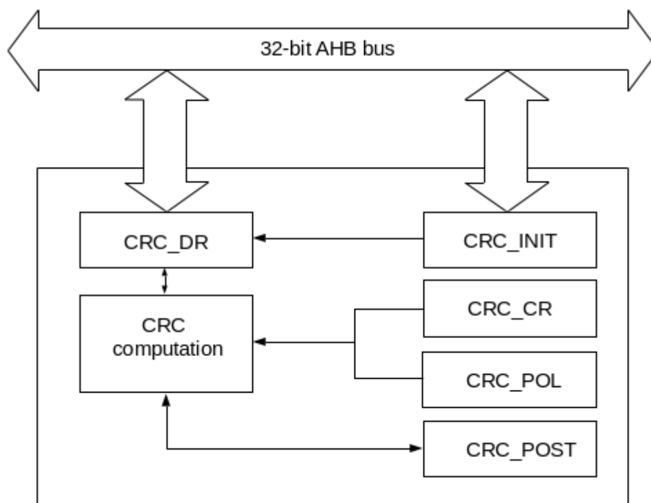
Рисунок 14.1 – Структура блока проверки подсчётом циклически избыточным кодом
