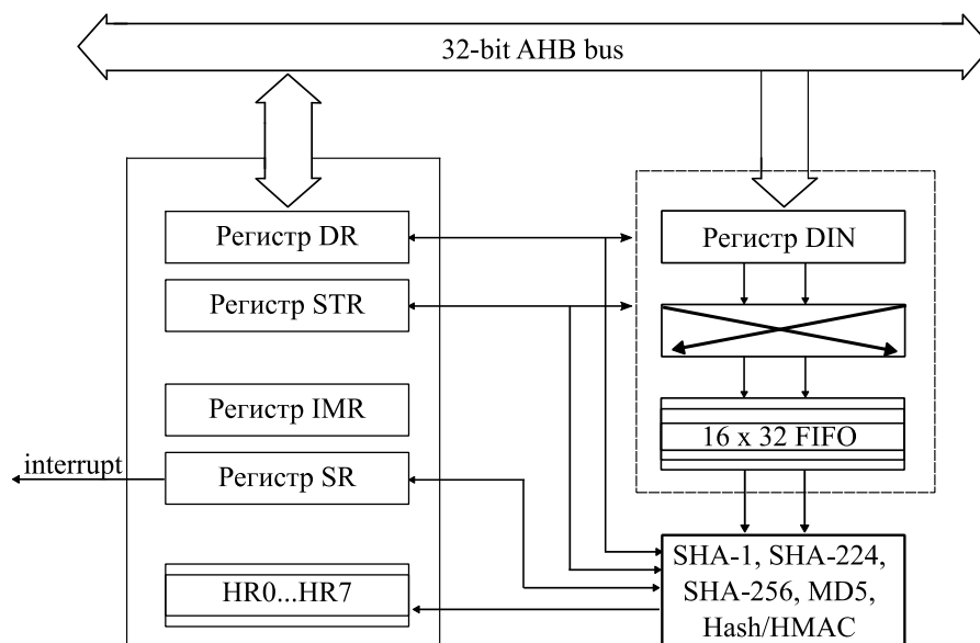
Рисунок 15.1 - Блок схема хеш-процессора
