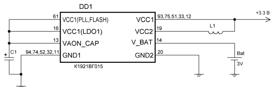
Рисунок 5.3 – Пример схемы подключения питания с высоким потреблением от V_BAT
