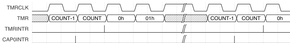
Рисунок 13.3 — Установка флагов прерываний в режиме «вверх»
