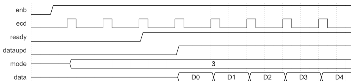
Рисунок 22.4 – Диаграмма переключения внутренних сигналов в режиме 3.
