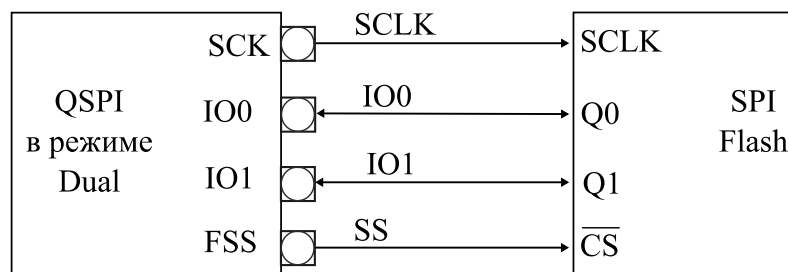
Рисунок 28.4 – Подключение внешней flash-памяти в режиме dual QSPI
