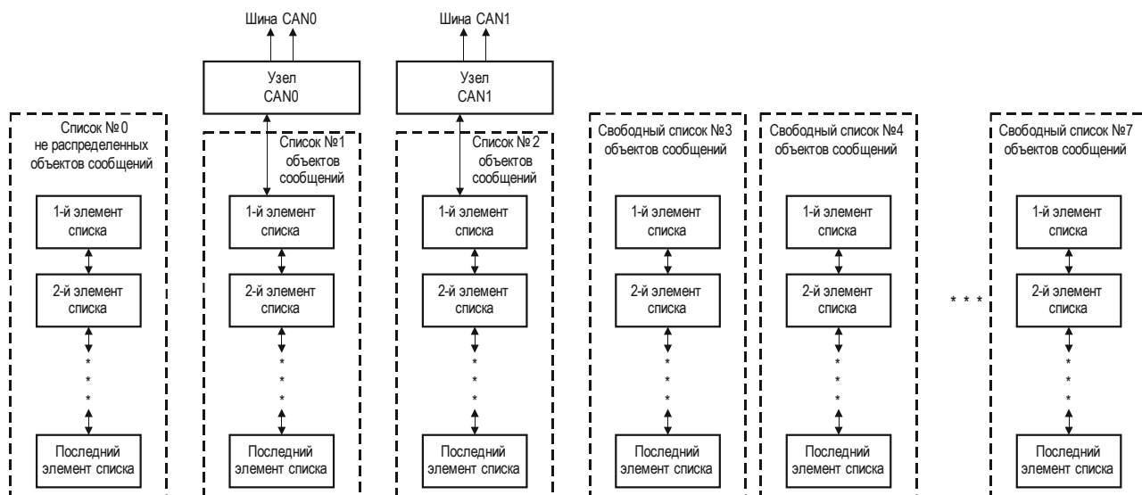
Рисунок 26.17 – Списки контроллера CAN
