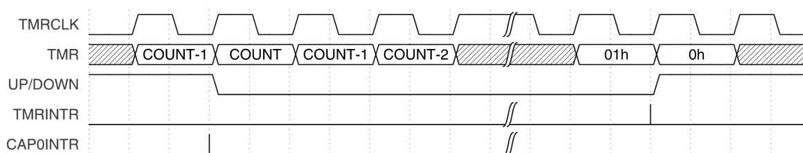
Рисунок 12.8 – Установка флагов прерываний в режиме «вверх/вниз»
