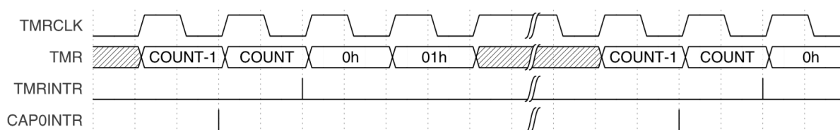
Рисунок 12.3 — Установка флагов прерываний в режиме «вверх»
