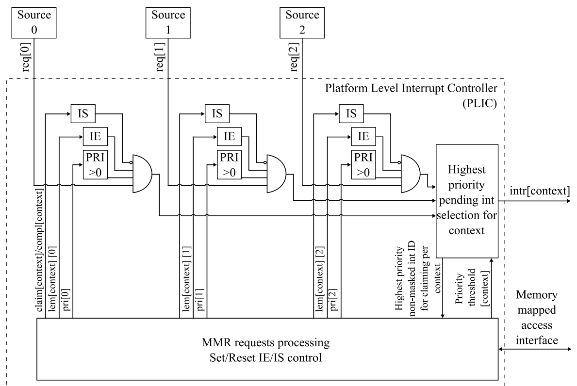
Рисунок 9.1 – Структурная схема PLIC
