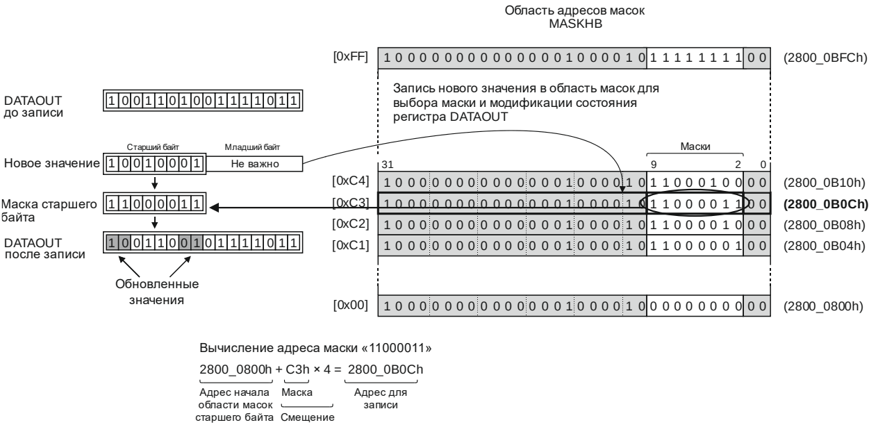
Рисунок 11.5 – Механизм изменения состояния старшего байта порта А с маскированием
