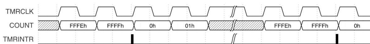
Рисунок 13.5 — Установка флага прерываний в непрерывном режиме
