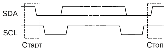
Рисунок 27.2 – Состояния старта и стопа
