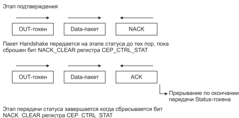
Рисунок 30.5 – Подтверждение
