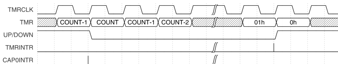
Рисунок 13.8 – Установка флагов прерываний в режиме «вверх/вниз»
