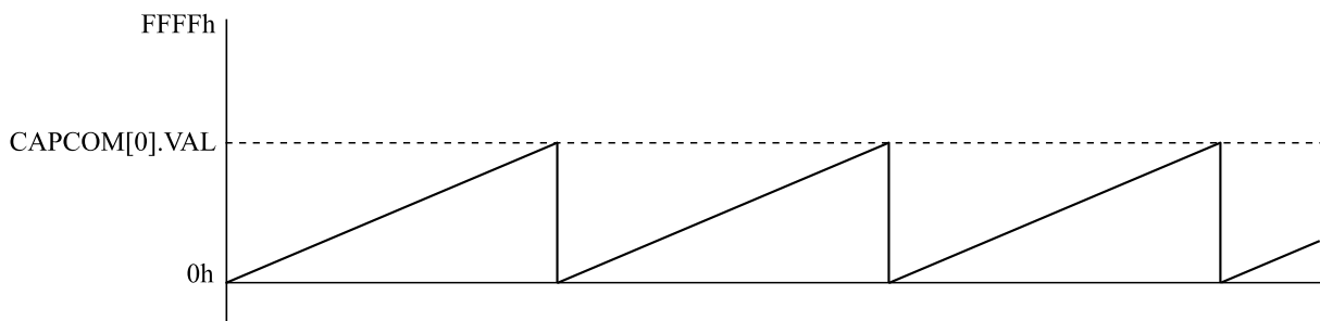
Рисунок 13.2 — Режим «вверх»
