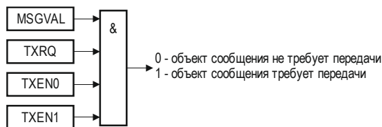
Рисунок 26.21 – Формирование запроса на передачу объекта сообщения
