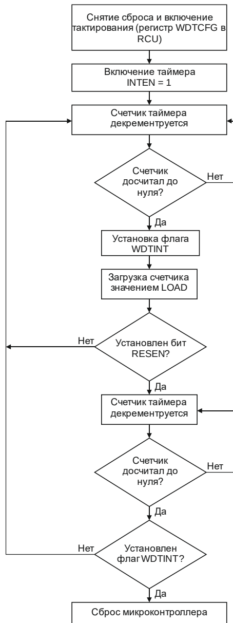
Рисунок 19.1 – Алгоритм работы сторожевого таймера
