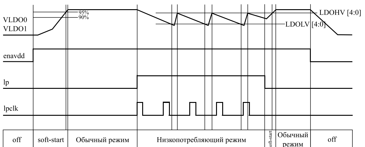
Рисунок 5.4 – Диаграмма работы регуляторов в режиме пониженного потребления
