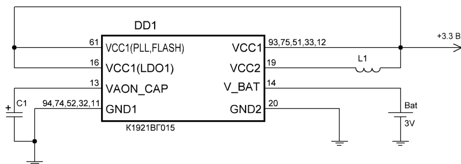
Рисунок 5.2 – Пример схемы подключения питания с низким потреблением от V_BAT
