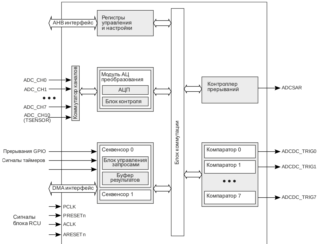
Рисунок 21.1 – Структурная схема блока АЦП
