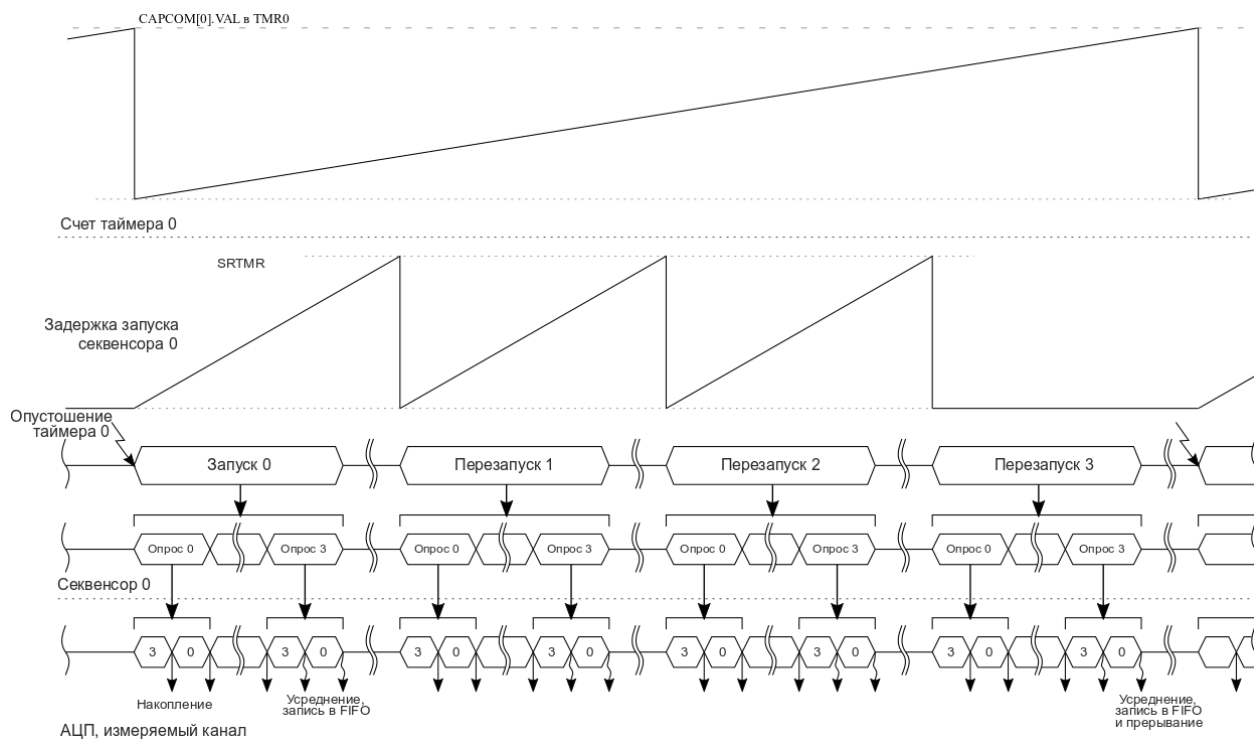
Рисунок 21.21 – Диаграммы равномерно распределенных измерений по периоду таймера
