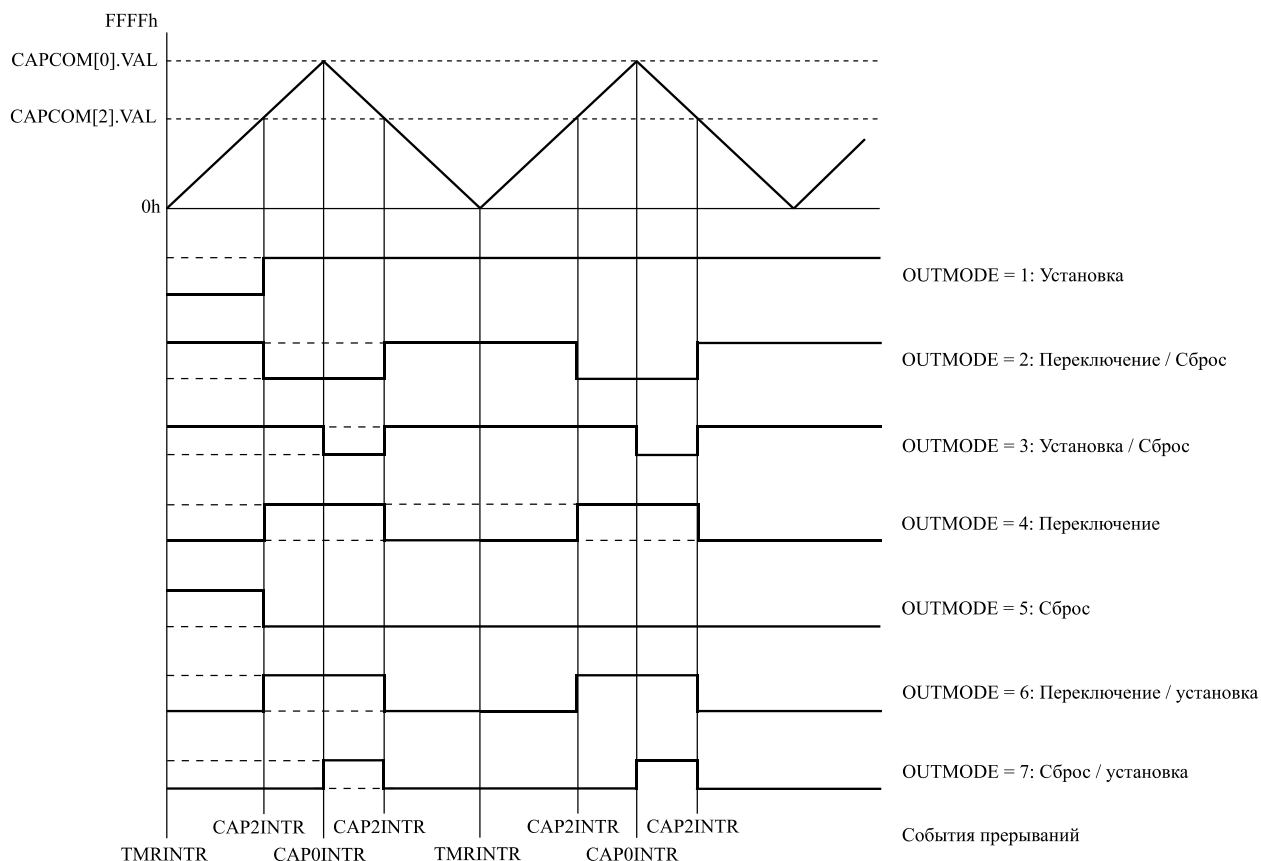
Рисунок 13.14 – Таймер в режиме счета «вверх/вниз» (пример вывода)
