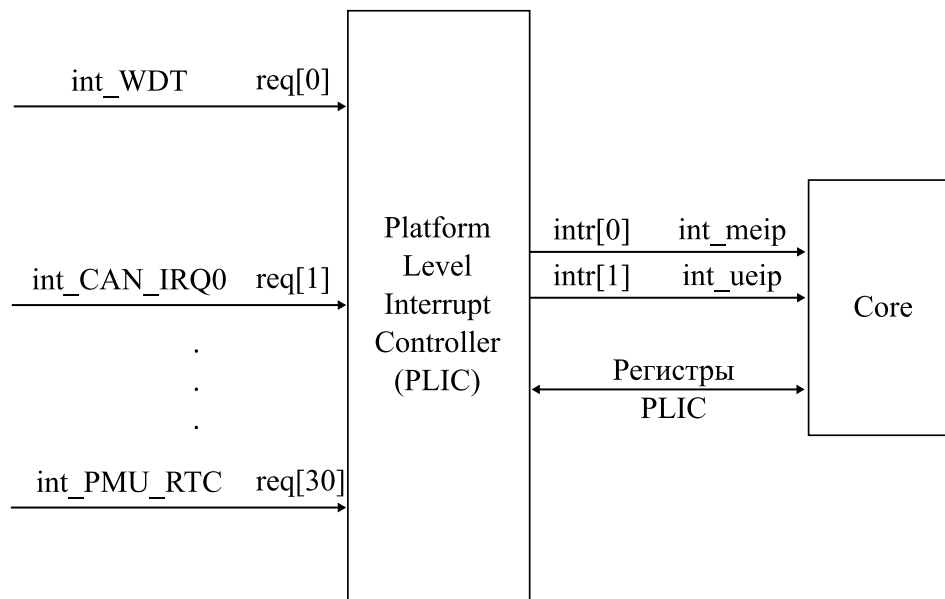
Рисунок 9.1 – Структурная схема контроллера обработки внешних прерываний
