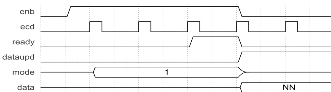
Рисунок 22.2 – Диаграмма переключения внутренних сигналов в режиме 1.
