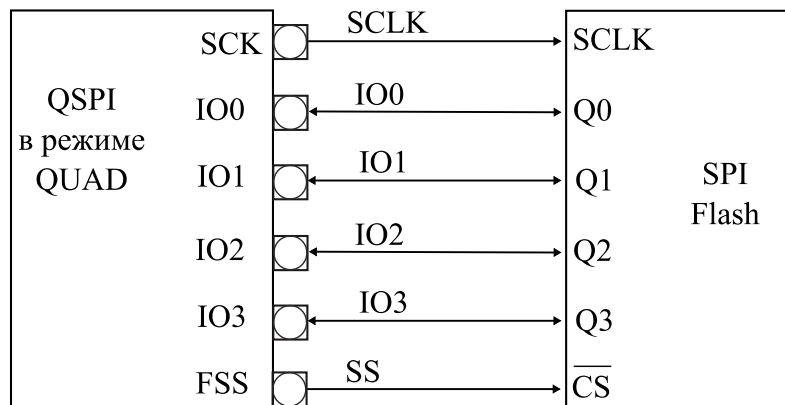
Рисунок 28.5 – Подключение внешней flash-памяти в режиме quad QSPI
