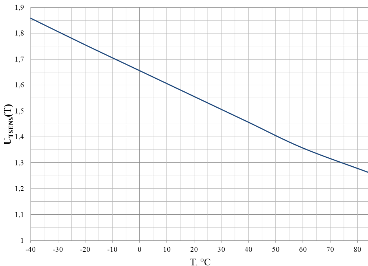
Рисунок 23.3 – График зависимости напряжения на выходе датчика от температуры при использовании внутреннего источника тока опорного напряжения ADCSD
