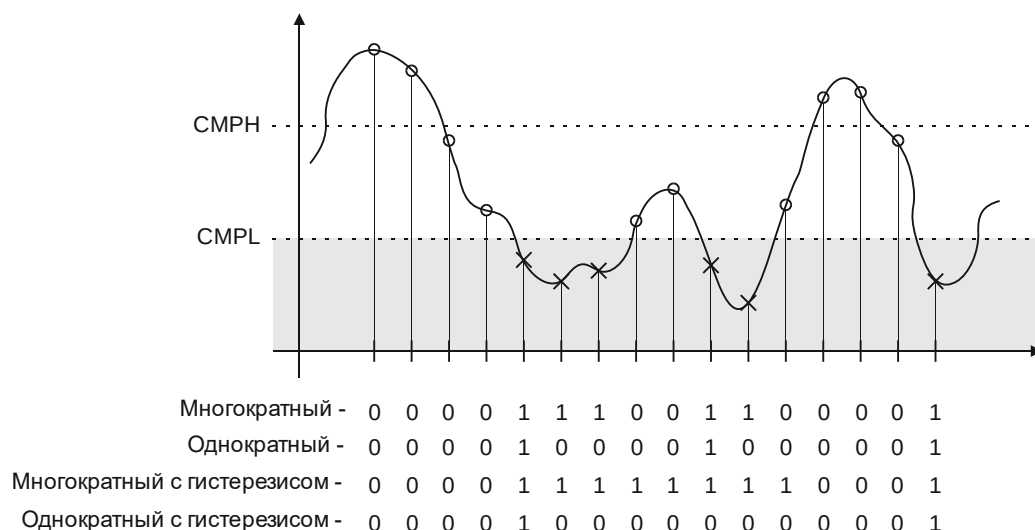
Рисунок 21.15 – Функционирование триггера при CTC = 00b
