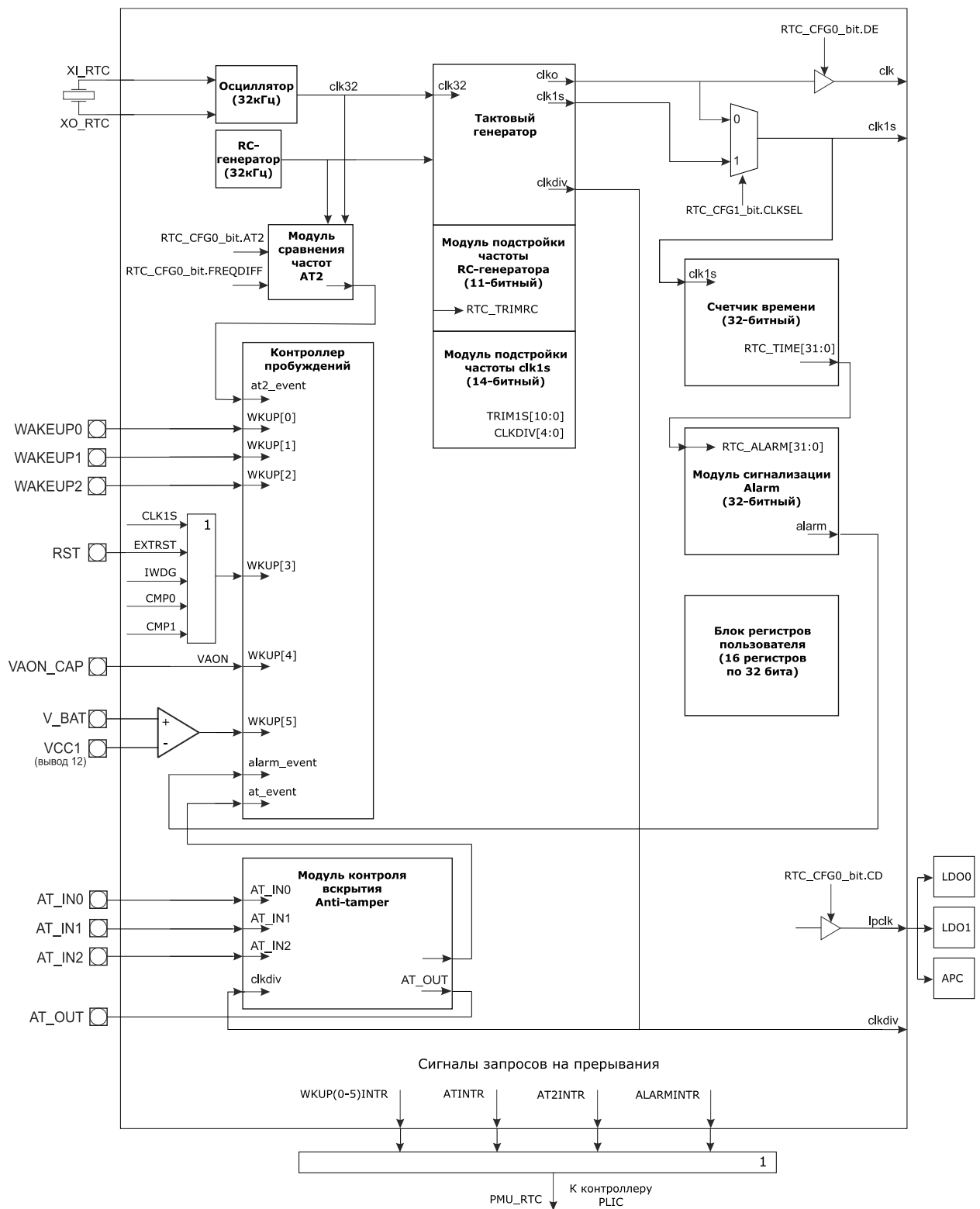
Рисунок 18.1 – Структура блока RTC
