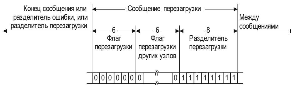
Рисунок 26.6 – Сообщение о резервации
