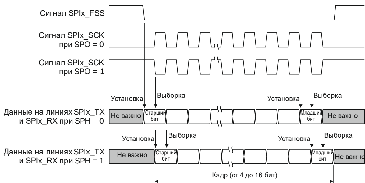
Рисунок 29.4 – Передача кадров данных в интерфейсе SPI
