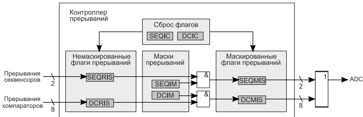
Рисунок 21.18 – Контроллер прерываний
