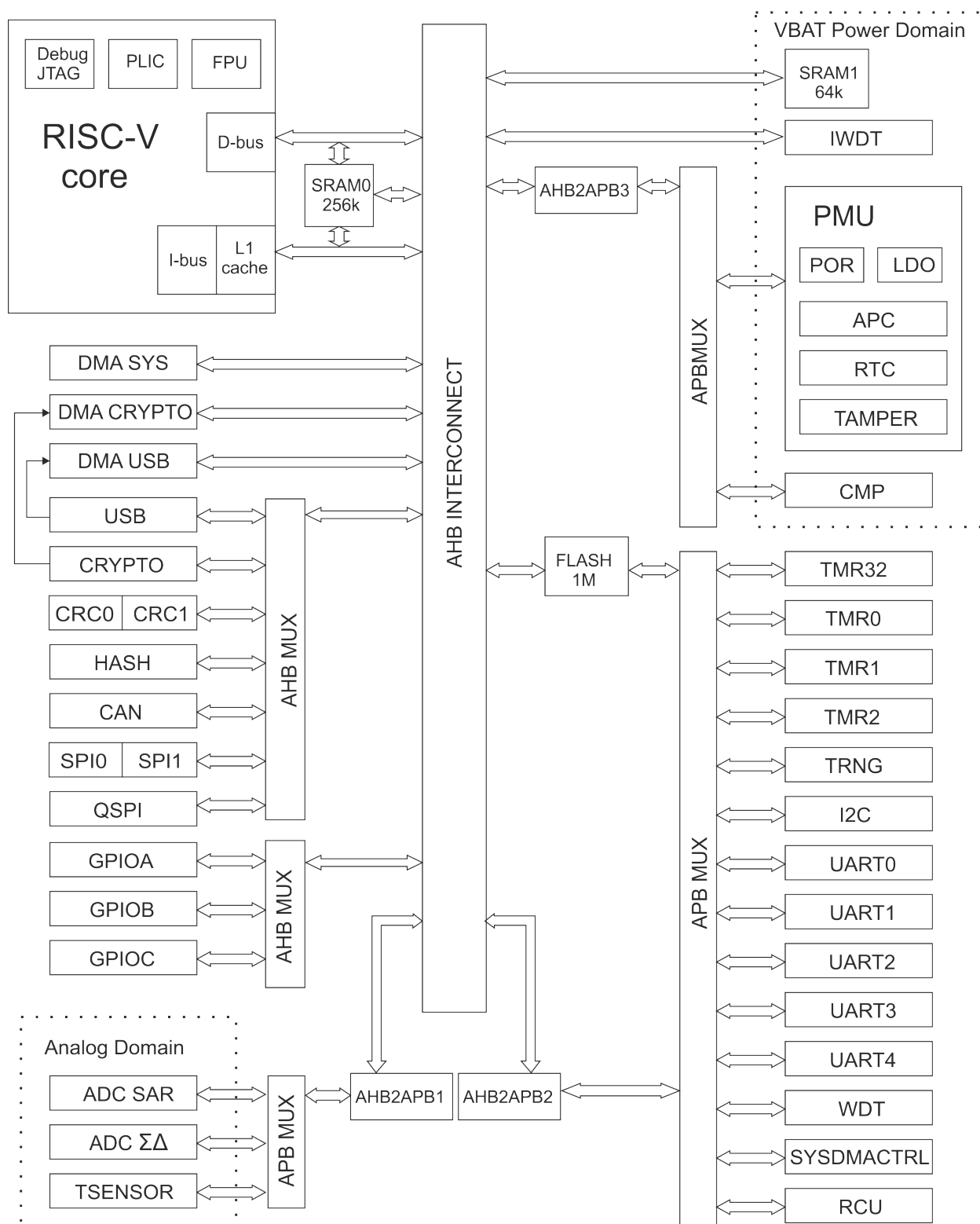
Рисунок 2.1 – Структурная схема микроконтроллера
