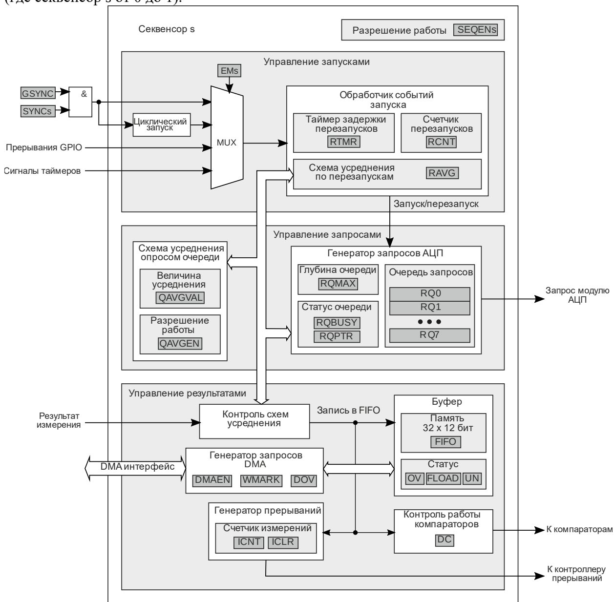
Рисунок 21.2 – Структурная схема секвенсора
