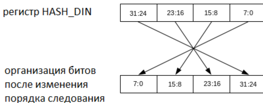
Рисунок 15.3 – Представление входных данных как байтов
