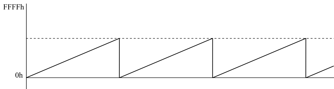
Рисунок 13.4 — Непрерывный режим
