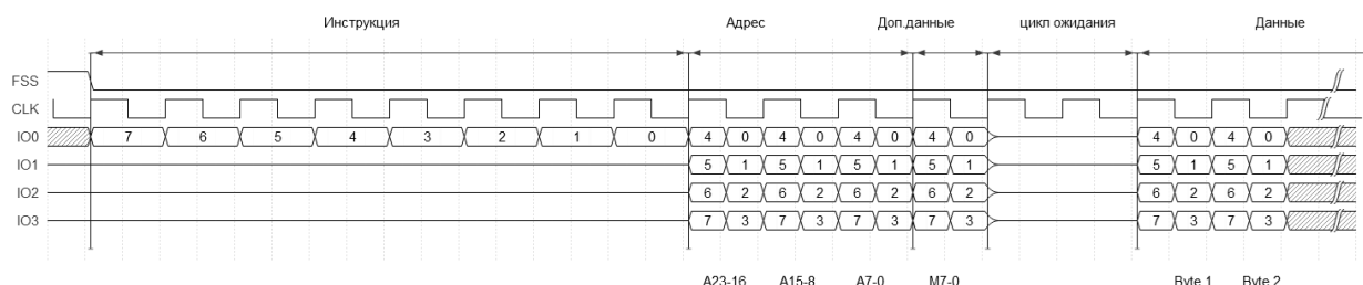
Рисунок 28.6 – Пример передачи команды DDR в режиме передачи данных по четырем линиям
