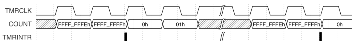
Рисунок 12.5 — Установка флага прерываний в непрерывном режиме
