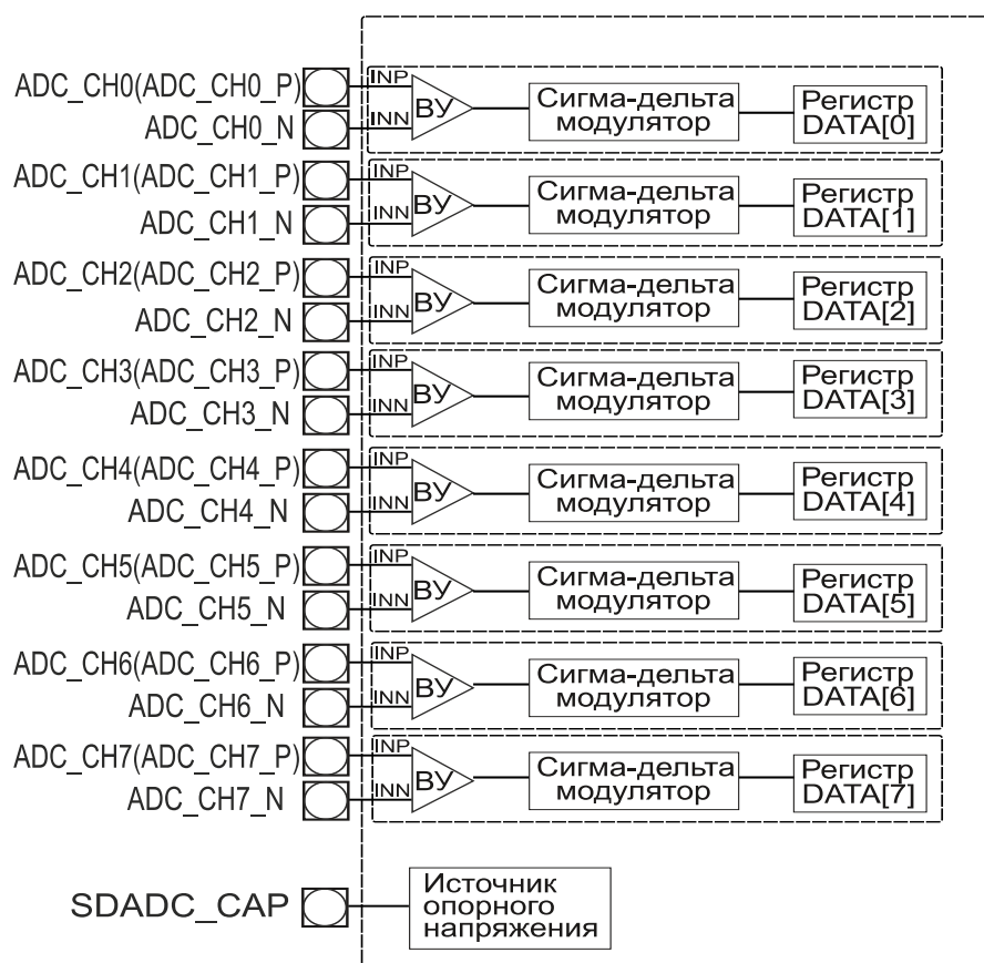
Рисунок 22.1 – Структурная схема сигма-дельта АЦП
