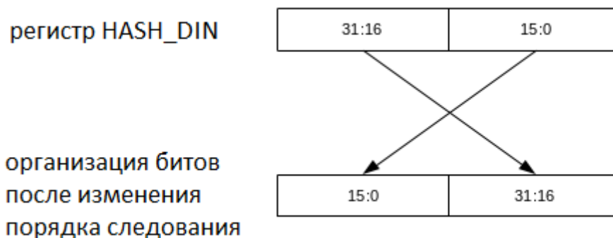
Рисунок 15.4 – Представление входных данных как полуслов
