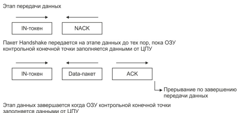
Рисунок 30.4 – Передача данных
