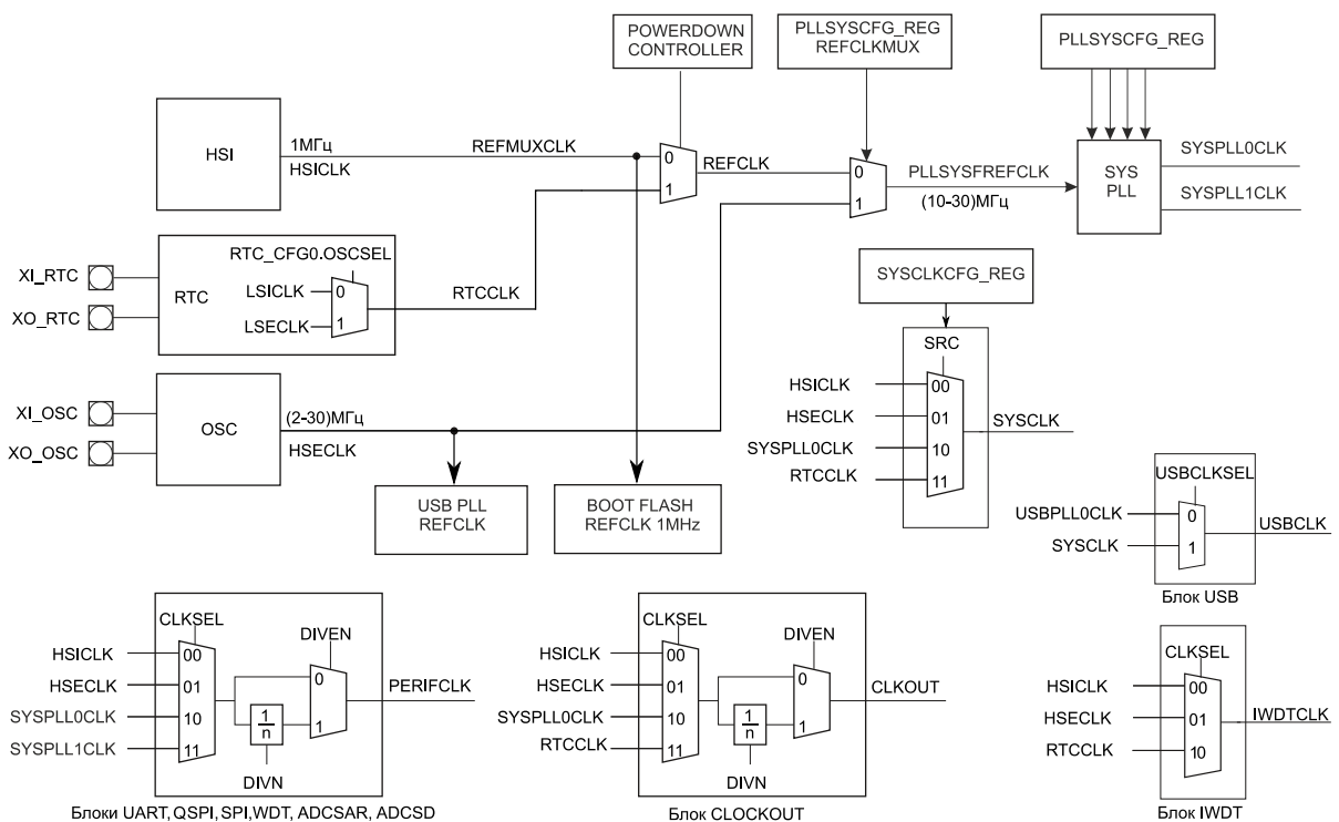
Рисунок 4.1 – Схема синхронизации
