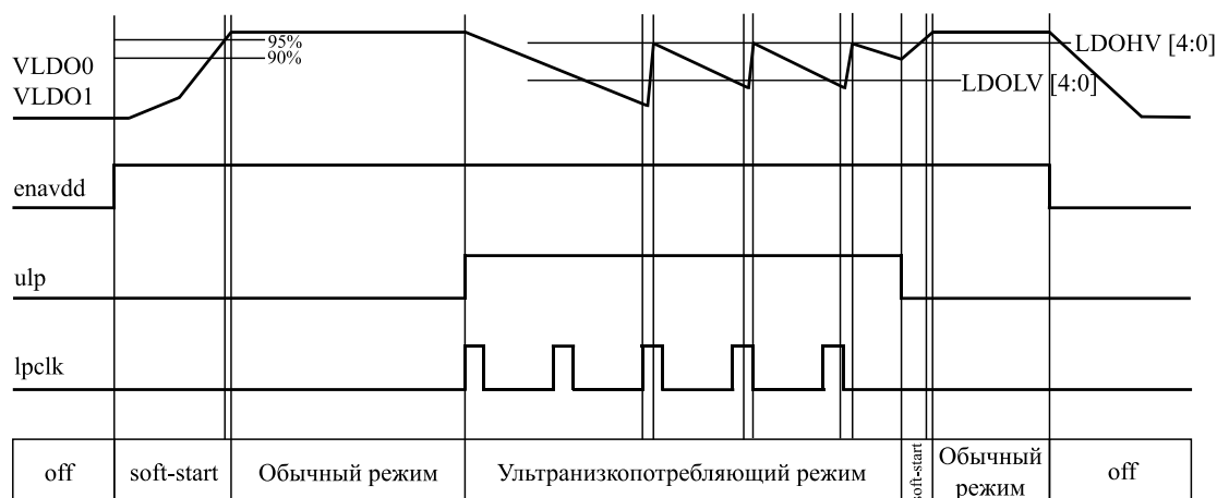
Рисунок 5.5 – Диаграмма работы регуляторов в режиме ультранизкого потребления
