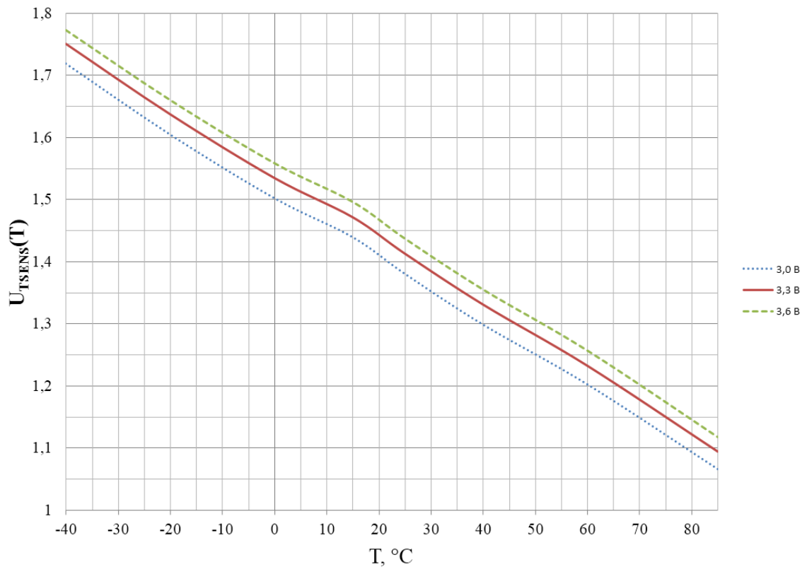
Рисунок 23.2 – График зависимости напряжения на выходе датчика от температуры при использовании внутреннего источника тока
