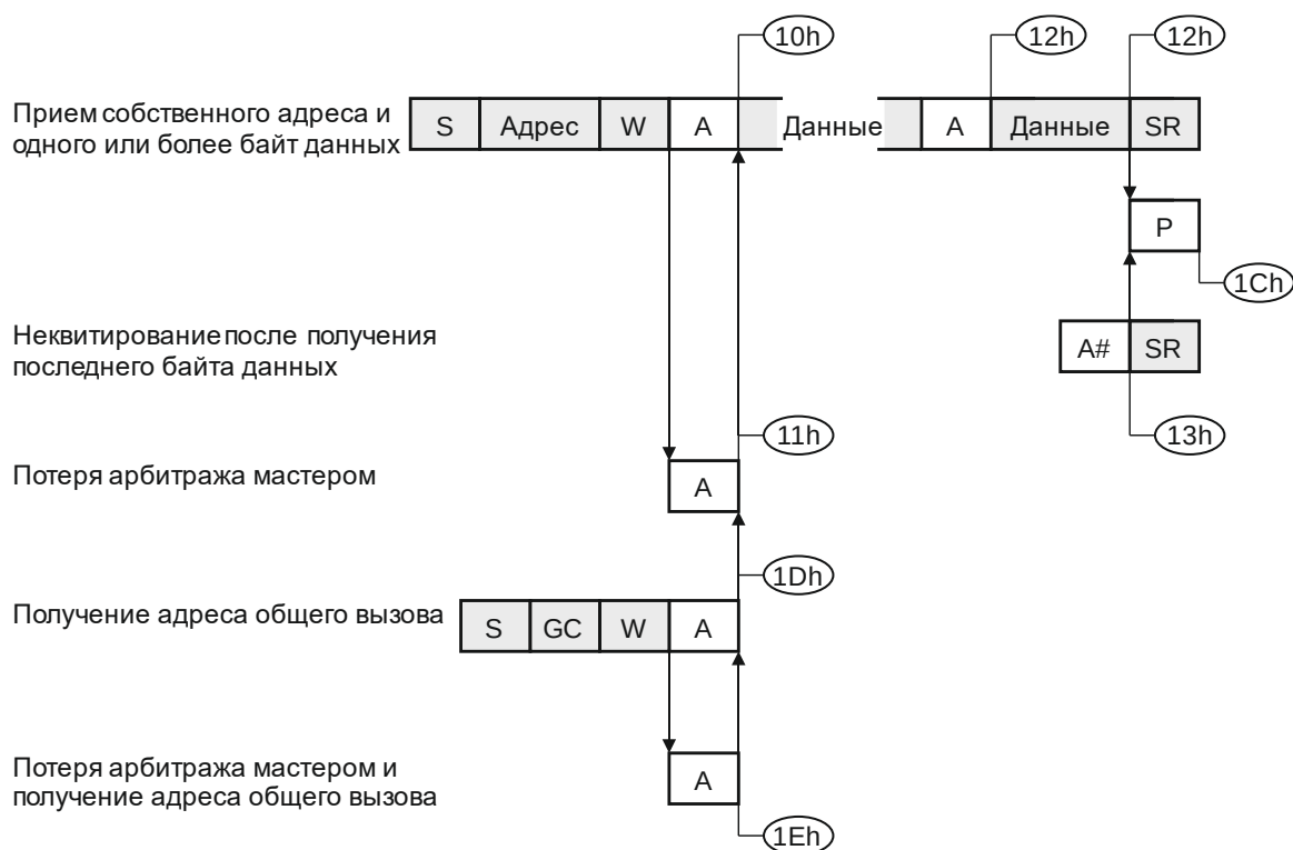
Рисунок 26.20 – Режим FS ведомого приемника
