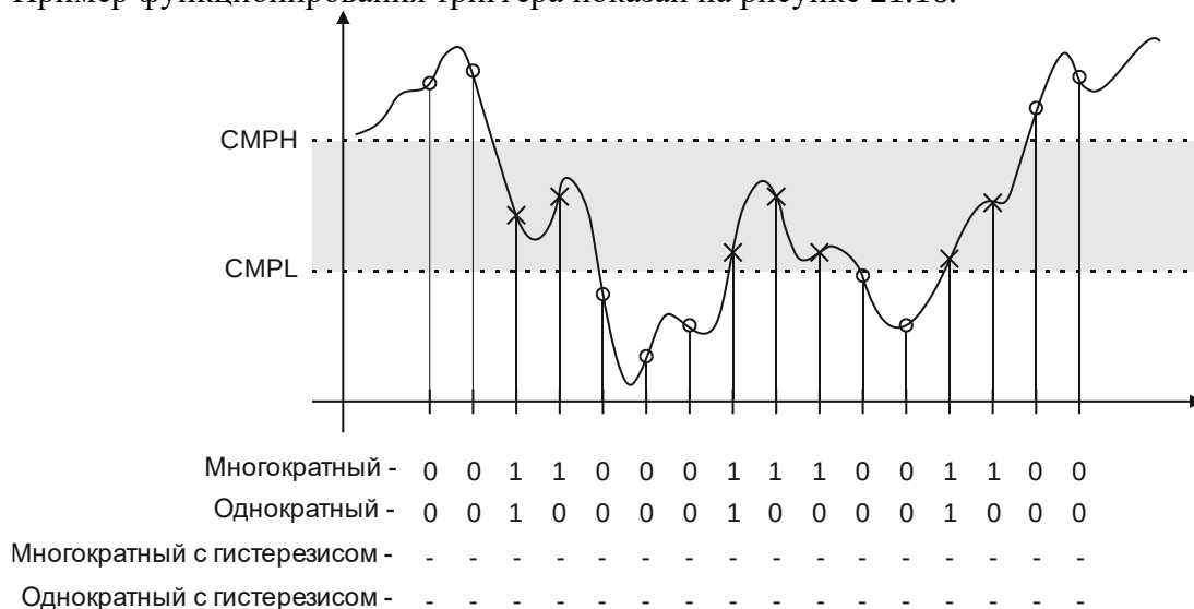
Рисунок 21.16 – Функционирование триггера при СТС = 01b
