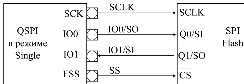
Рисунок 28.3 – Подключение внешней flash-памяти в режиме single QSPI
