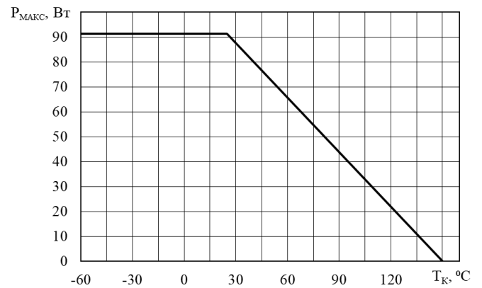
Рисунок 10 - Зависимость предельной мощности
