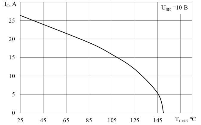
Рисунок 14 – Типовая зависимость предельного постоянного тока стока
