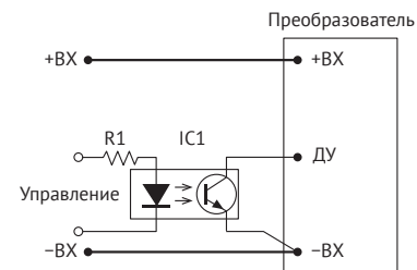
Рис. 7. «ДУ» с помощью оптрона.
