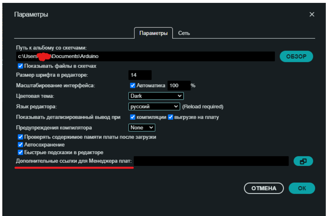
Рисунок 5 – Меню «Параметры»
