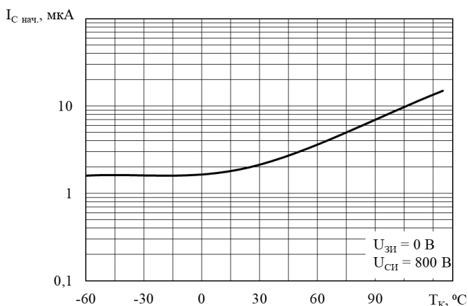
Рисунок 11 - Типовая зависимость начального тока стока
