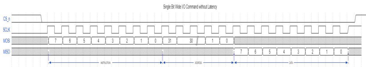
Рисунок 65 – Временная диаграмма инструкции с данными без адреса
