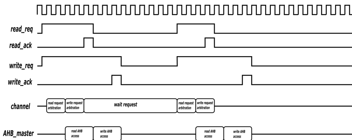
Рисунок 5 – Временная диаграмма длительности доступа к шине для одного канала с формированием сигнала снятия запроса
