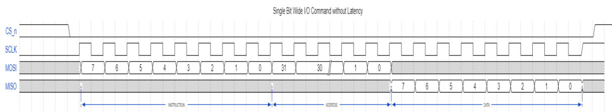
Рисунок 66 – Временная диаграмма инструкции с адресом и принимаемыми данными
