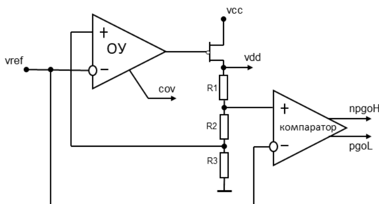
Рисунок 93 – Структурная схема регулятора напряжения
