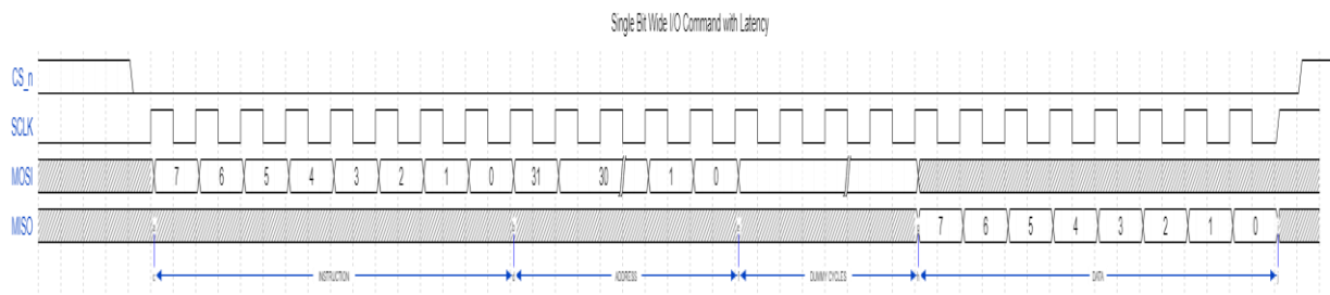
Рисунок 67 – Временная диаграмма инструкции с адресом и принимаемыми данными и задержкой
