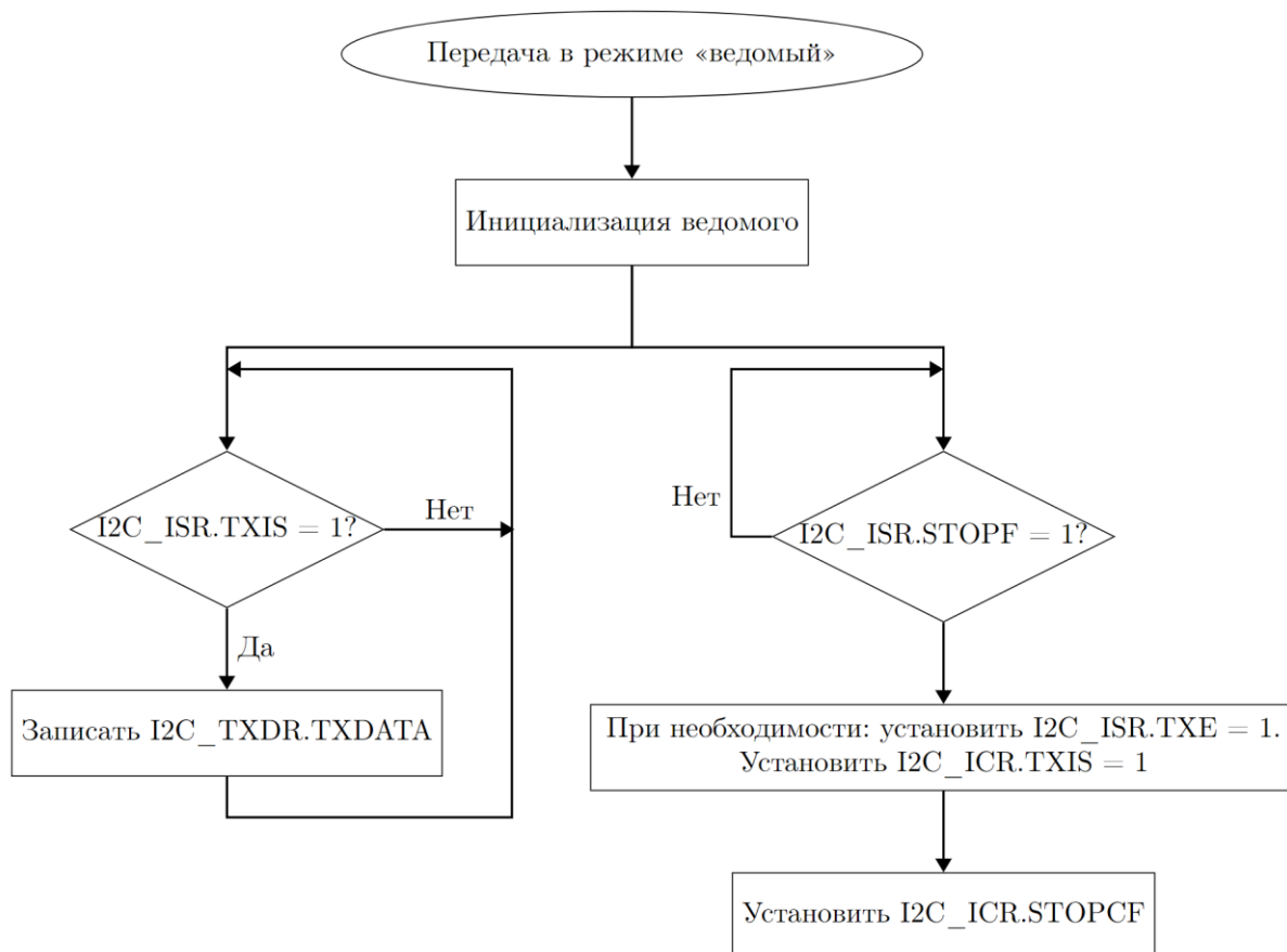
Рисунок 30 - Алгоритм передачи в режиме «ведомый», при NOSTRETCH=1
