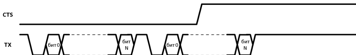
Рисунок 18 – Пример срабатывания сигнала, запрещающего передачу (CTS=1)
