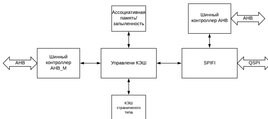
Рисунок 58 – Общая структура контроллера
