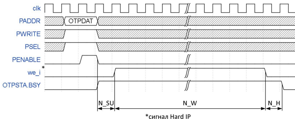
Рисунок 70 – Формы сигналов в процедуре записи
