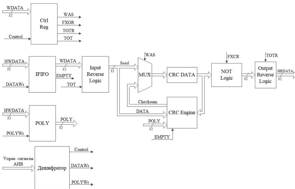
Рисунок 53 – Схема блока CRC
