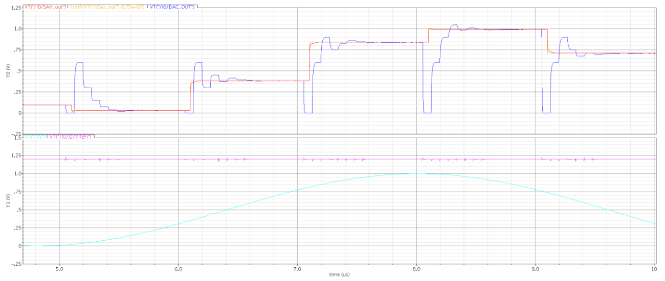
Рисунок 82 – Временные диаграммы работы АЦП
