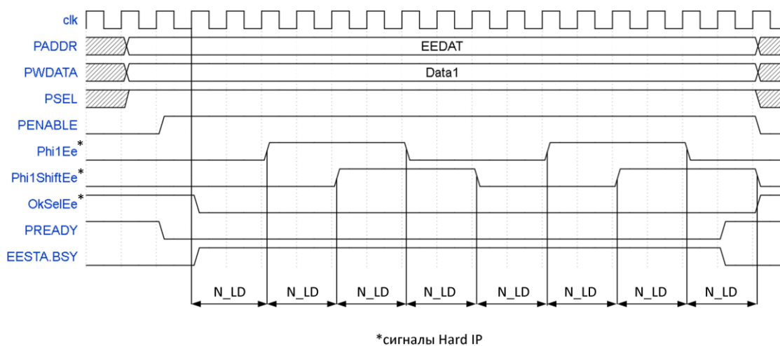
Рисунок 73 – Формы сигналов в процедуре заполнения буфера записи
