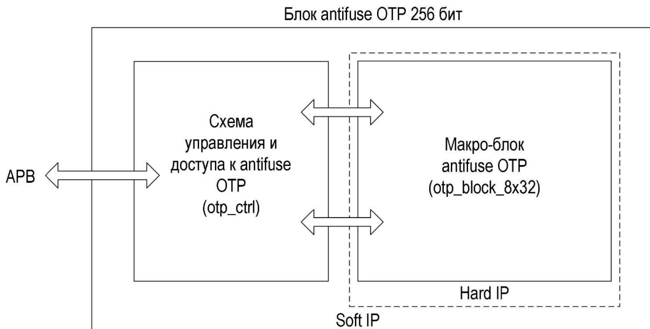
Рисунок 69 – Схема блока OTP
