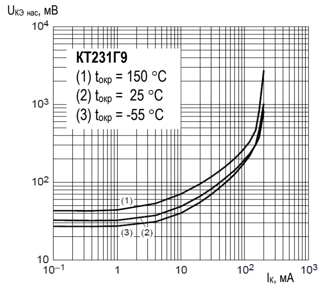
Рис.1 Типовая зависимость напряжения насыщения коллектор-эмиттер от тока коллектора транзисторов (при I_{к} / I_{Б} = 20 )
