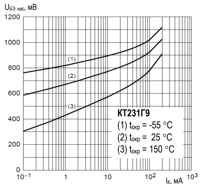
Рис.2 Типовая зависимость напряжения насыщения база-эмиттер от тока коллектора транзисторов (при I_{к} / I_{Б} = 10 )
