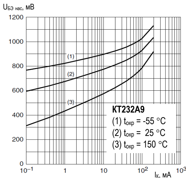
Рис.2 Типовая зависимость напряжения насыщения база-эмиттер от тока коллектора транзисторов (при I_{к} / I_{Б} = 10 )
